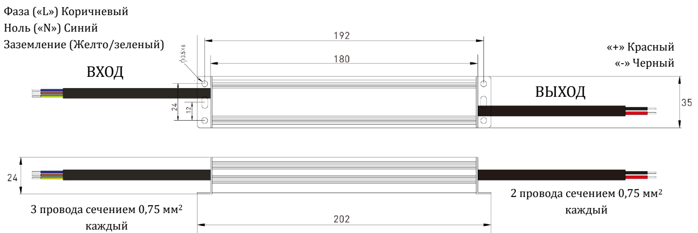
Рисунок 1 – Габаритные размеры и выводы источника питания
