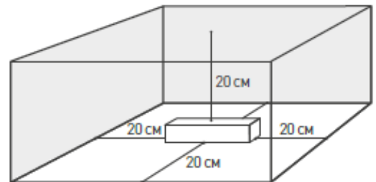
Рисунок 4 – Свободное пространство вокруг источника питания
